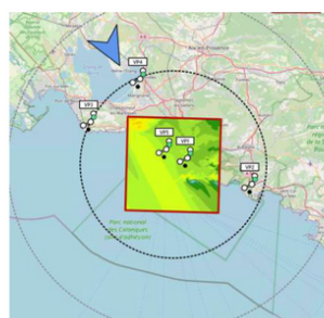
Carte du vent à 200m de hauteur pour les vents de NNO à l'échelle micro (25m de résolution en horizontal)
