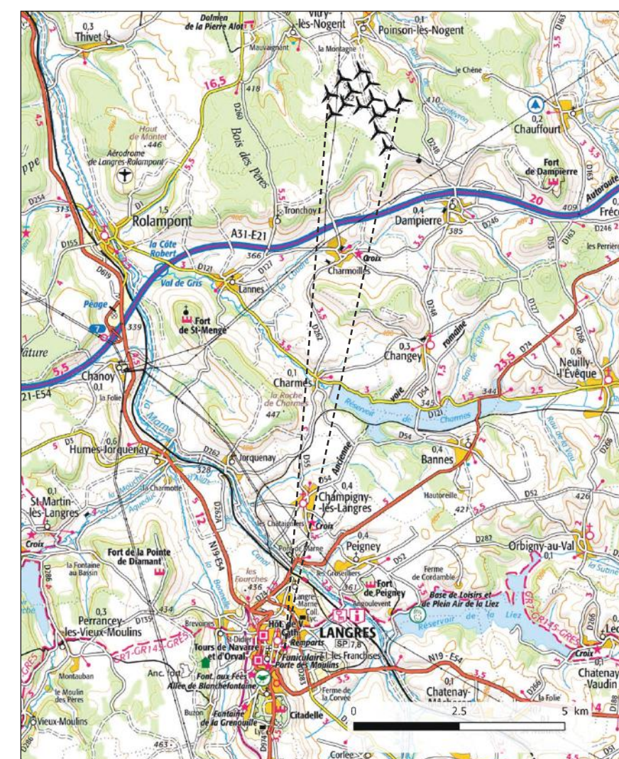
Fig. 7 : Implantation du parc éolien de Haut-de-Conge
